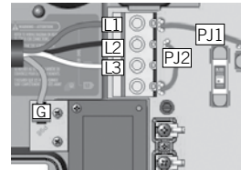
3-Phasen Delta (Kein Null-Leiter)
